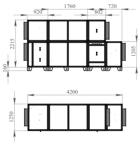
Правое исполнение
