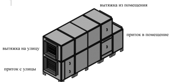
Правое исполнение
